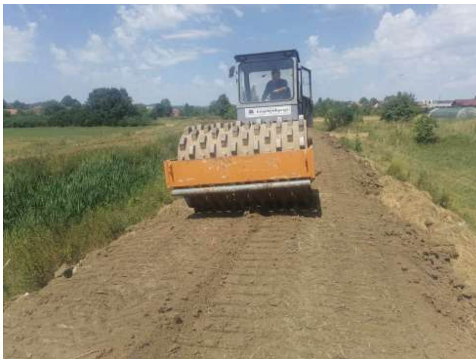
Надвишење левообалног насипа потока Бошњак
